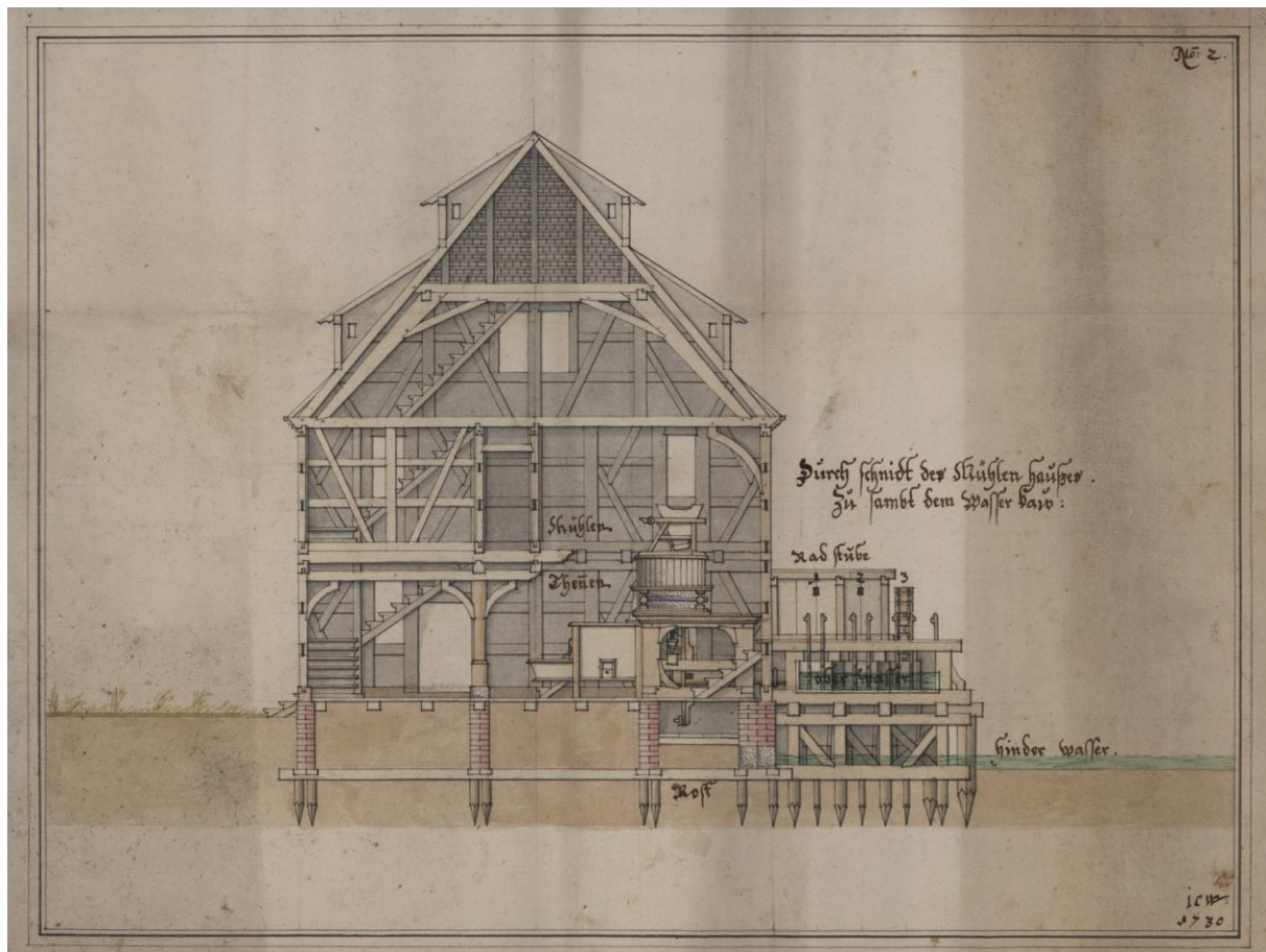
„Durschnitt“ eines Ulmer Muehlengebuedes, 1730 (StA Ulm, A[2082])
