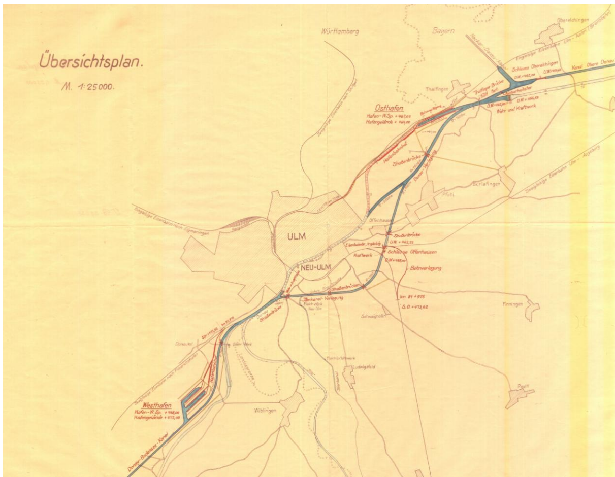
Entwurfsplan der Firma Grün & Bilfinger für das Ulmer Kanal- und Hafenprojekt 1932 (StA Ulm, B 660/50 Nr. 1/5).
