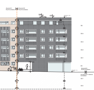
Strassenansicht Abschnitt B Südwest
