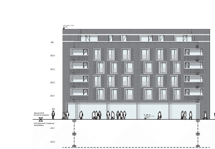
Platzansicht Abschnitt B Süd
