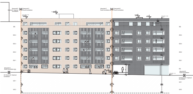
Straßenfassade Abschnitt C Südwest
