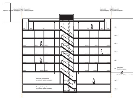
Schnitt Abschnitt C
