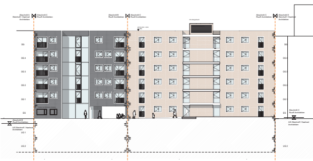
Hoffassade Abschnitt B
