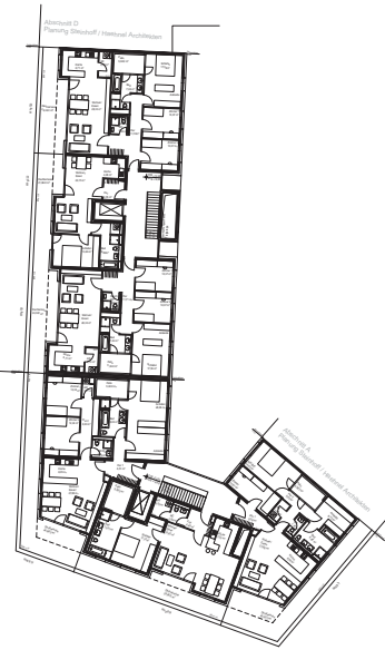
Dachgeschoss
