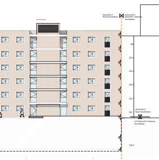
Hoffassade Abschnitt C Nordost
